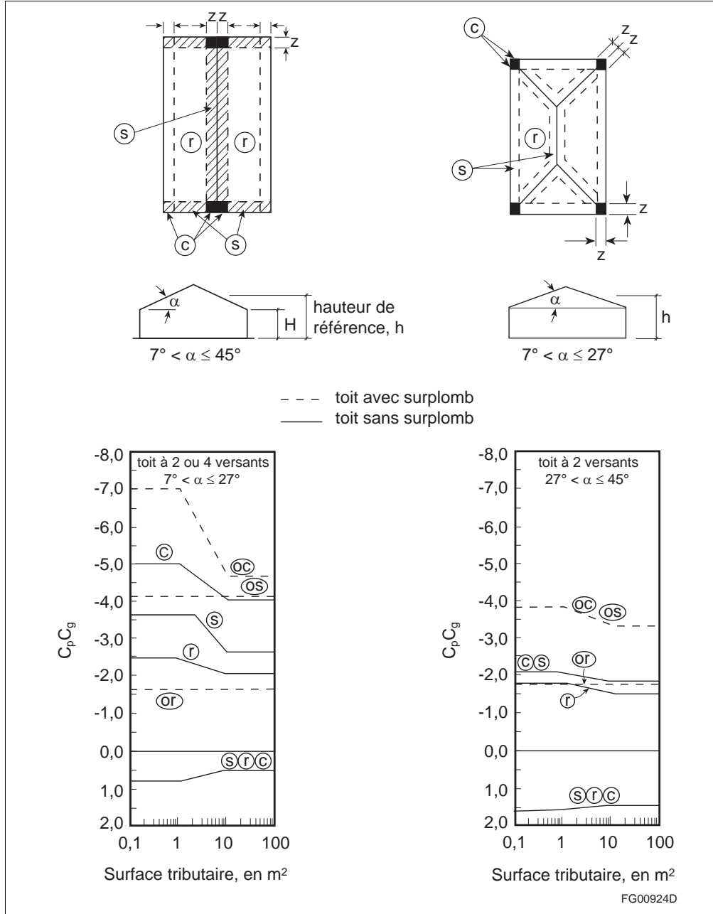
Figure 4.1.7.6.-E Valeurs extérieures de pointe du produit C_p C_g exercées sur un toit à 2 versants ou en croupe à portée simple dont la pente est supérieure à 7° pour le calcul des composants structuraux et du revêtement extérieur Faisant partie intégrante du paragraphe 4.1.7.6. 6)
