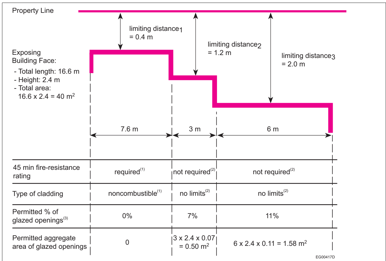
Figure A-9.10.15.4.(2)-A
