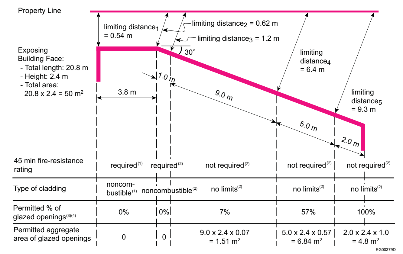
Figure A-9.10.15.4.(2)-C
