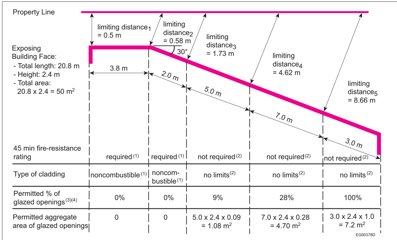
Figure A-9.10.15.4.(2)-B
